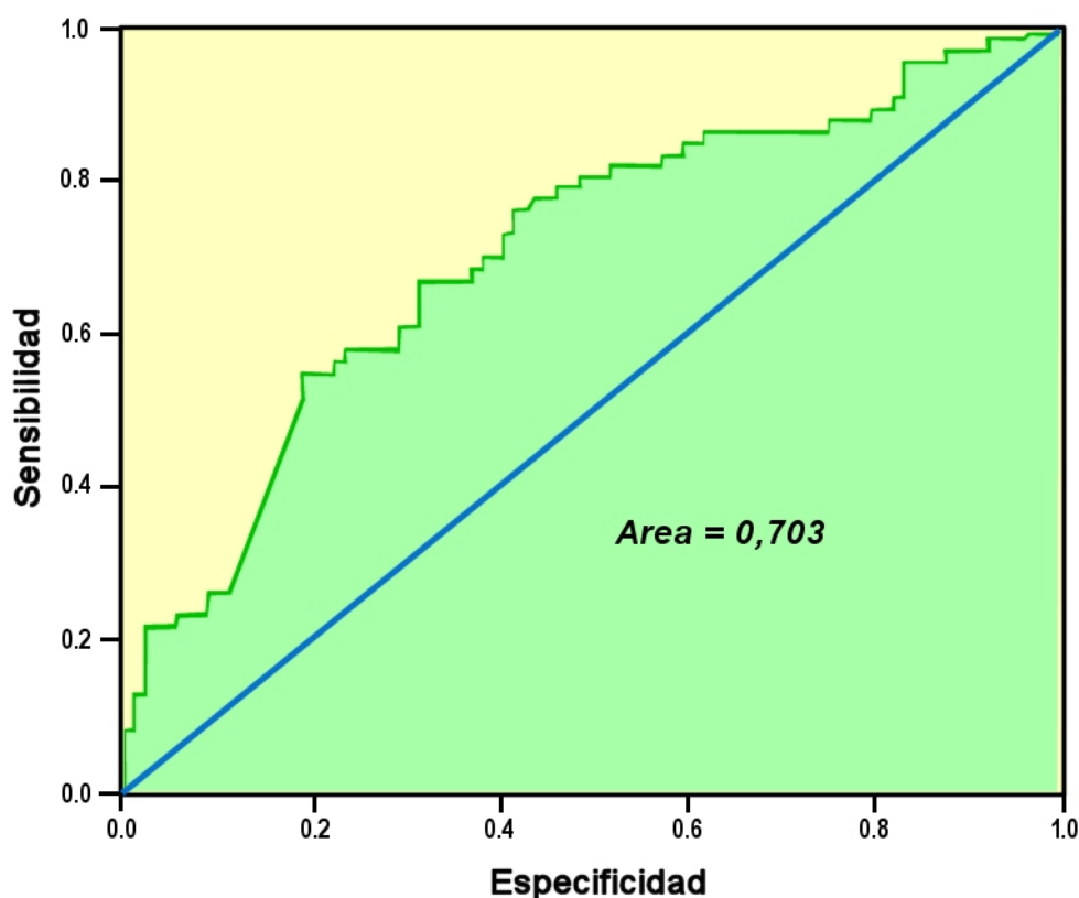
Gráfico 15 - Curva COR de la variable «% no clínico» (los segmentos diagonales son producidos por los empates)
