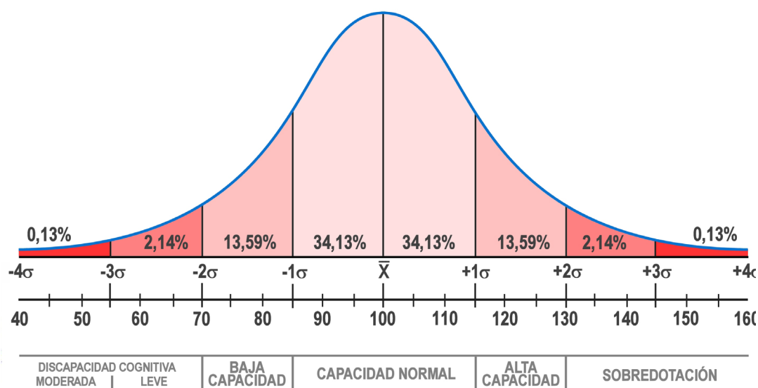
Gráfico 6 - Curva de Gauss de distribución de la inteligencia en la población
